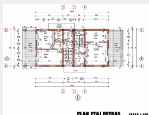
PLAN ETAJ RETRAS
